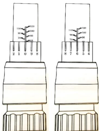
Przykład 1: 60Nm
