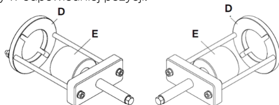
Ustawienie pierścienia oporowego w zależności od strony zależności od obsługiwanego pojazdu.
